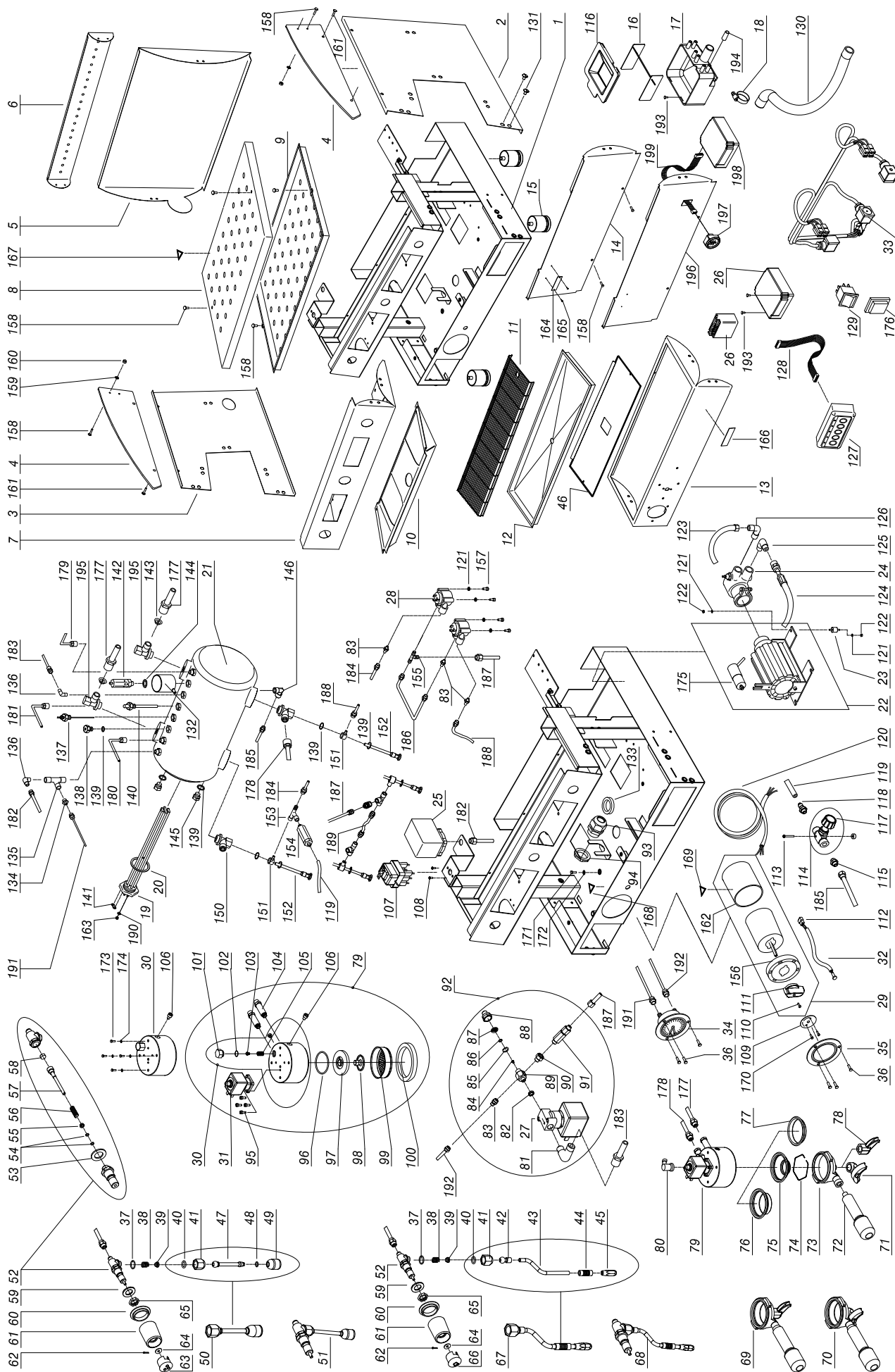
Esploso modello CAPRI DELUXE agg. 02-09
